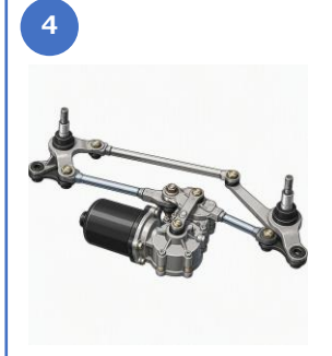
4 ワイパー機構 モーターの回転をリンクへ伝え、ワイパーを往復駆動
