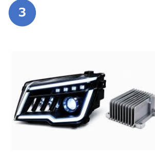
3 LEDライト用ヒートシンク LEDの発熱を放散し、光量と寿命の安定に寄与
