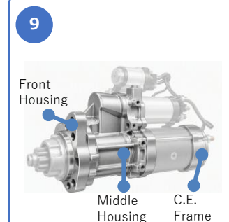
9 スタートASSY エンジンを始動し、クランクシャフト回転を伝達する電動ユニット
