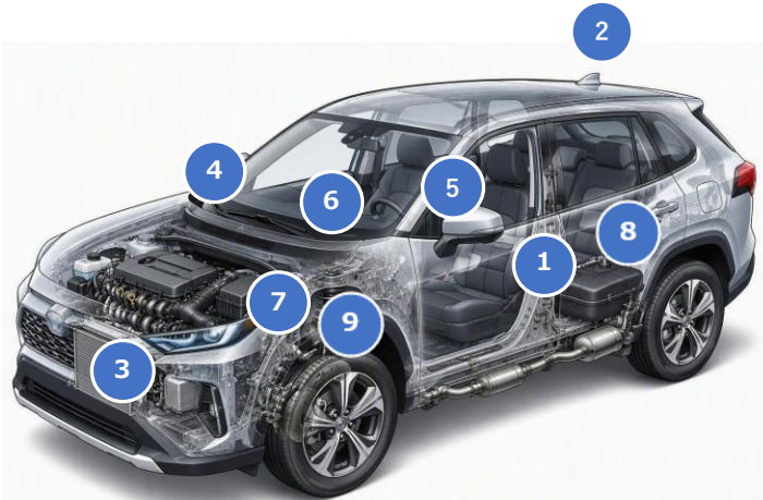
ICE車両 搭載位置
