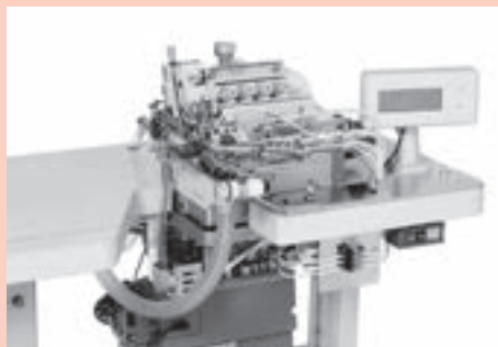
PHNシリーズ ●裾引きユニット
