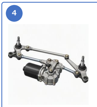
4 ワイパー機構 モーターの回転をリンクへ伝え、ワイパーを往復駆動
